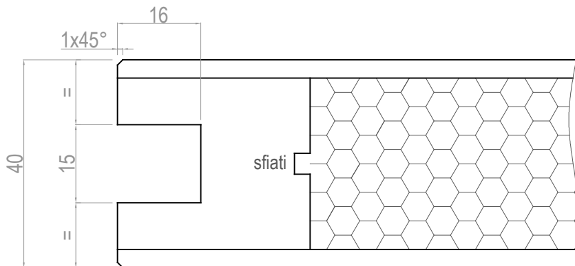
SEZIONE A-A LATI CORTI
